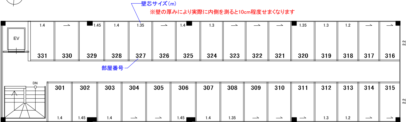
3階 平面図（31ルーム）
