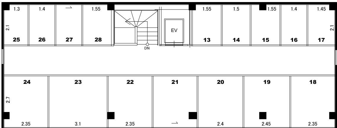
2階 平面図 (16ルーム)
