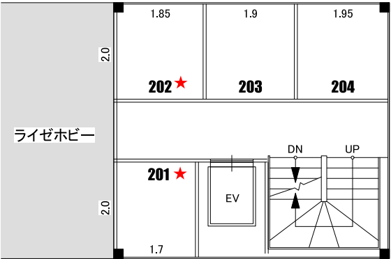
2階 平面図（4ルーム）
