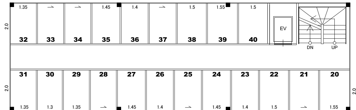
2階 平面図（21ルーム）
