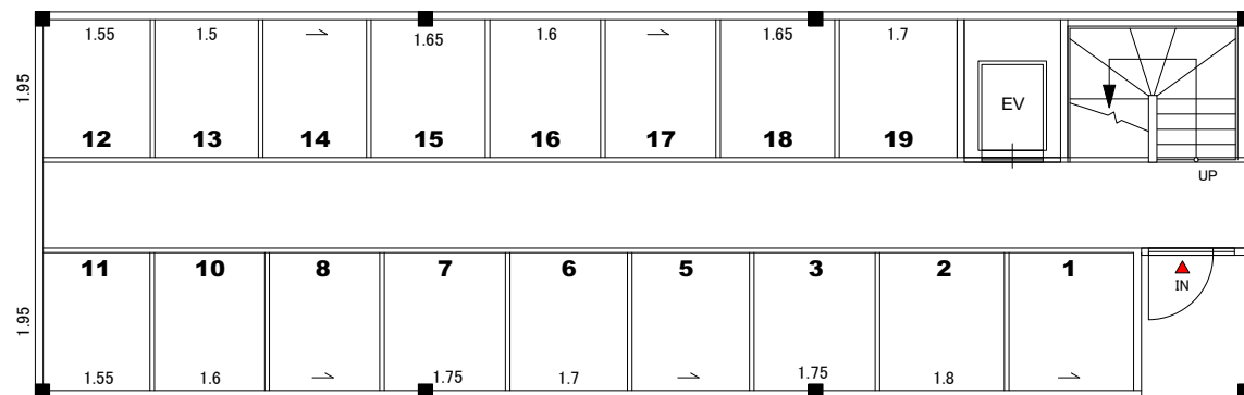
1階 平面図（17ルーム）
