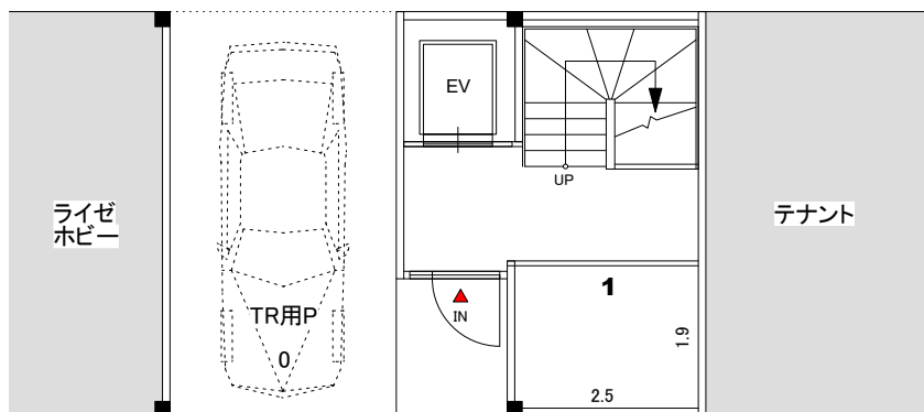
1階 平面図（1ルーム）
