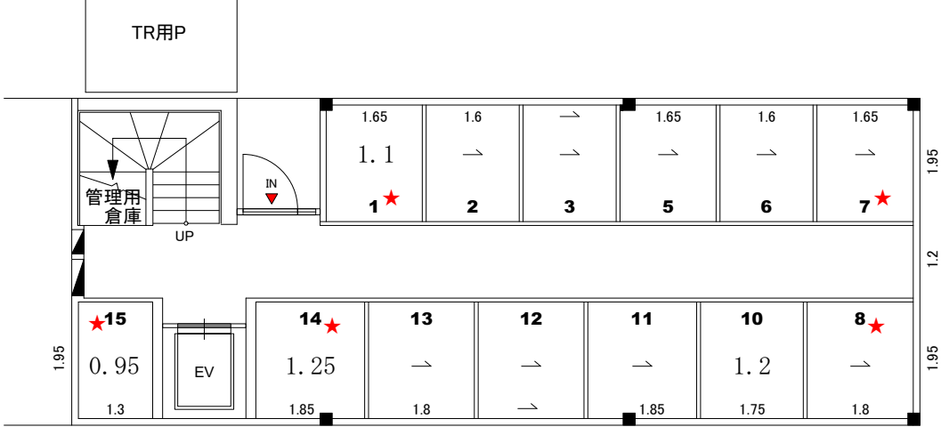
1階 平面図 (13ルーム)
