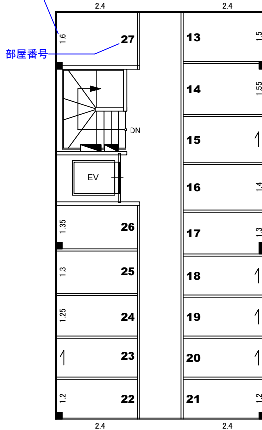
2階 平面図 (15ルーム)
