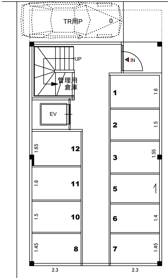
1階 平面図 (10ルーム)
